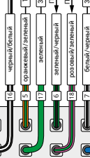
Разъем X8 (2-pin)
